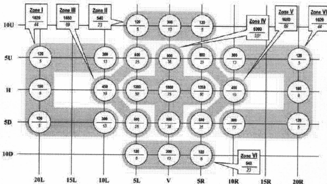
FIGURA 2- R/B – REQUISITOS FOTOMÉTRICOS CLASSE 2 – VERMELHO/AZUL
