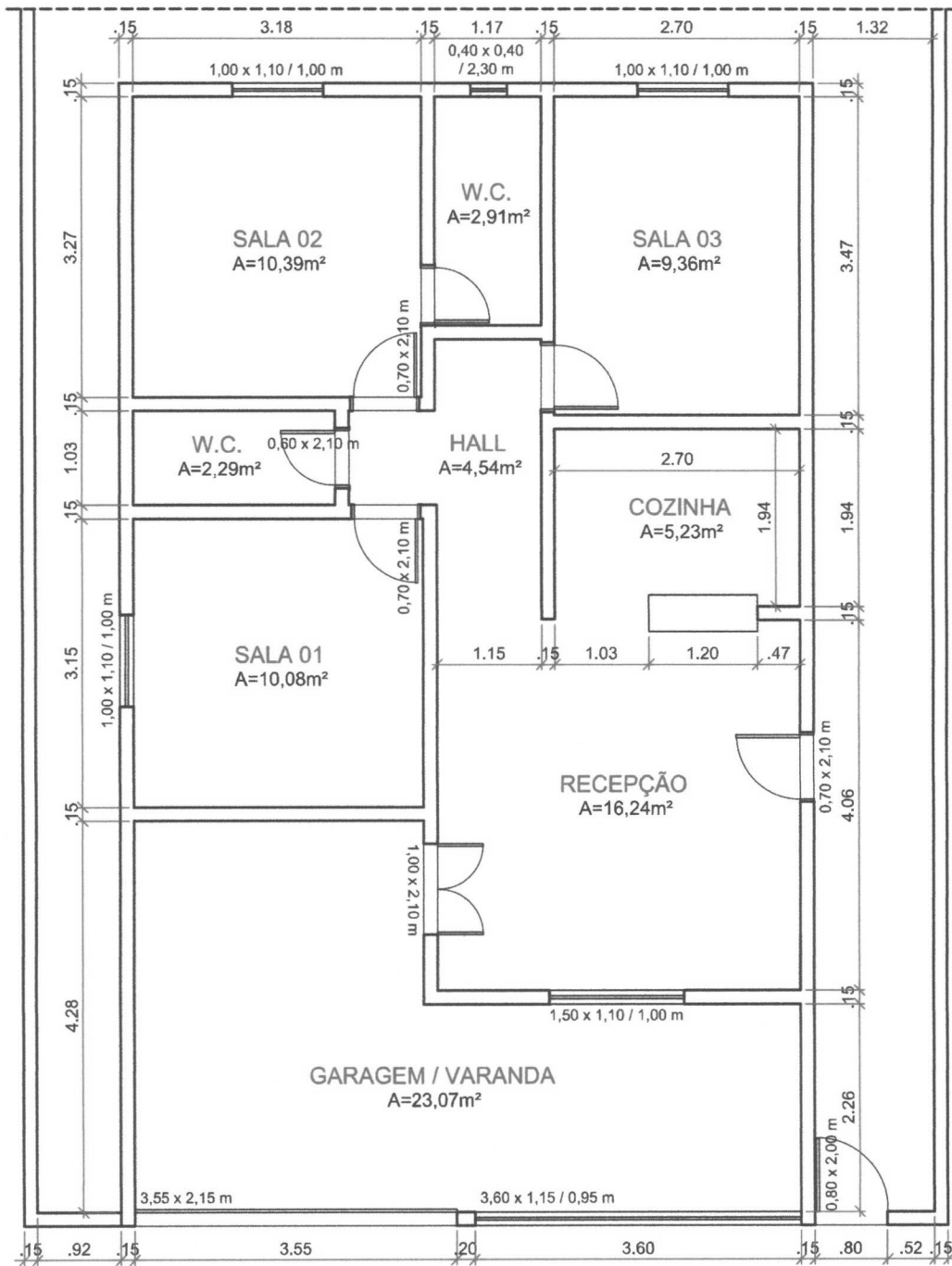
01 P.B. / DIRETORIAS DE MULHER E JUVENTUDE ESCALA: 1/75
