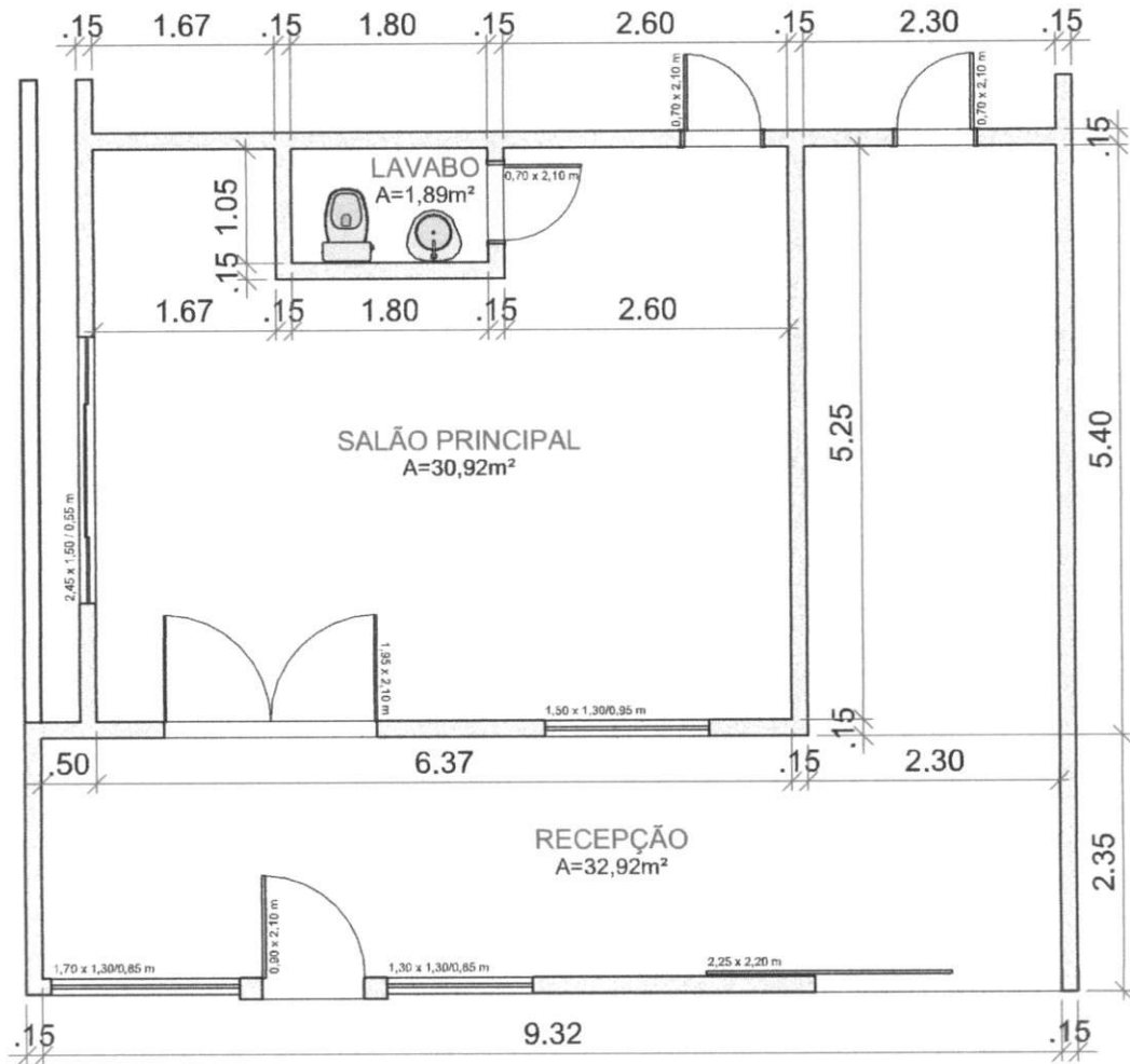
01 PLANTA - BAIXA ESCALA: 1/75
